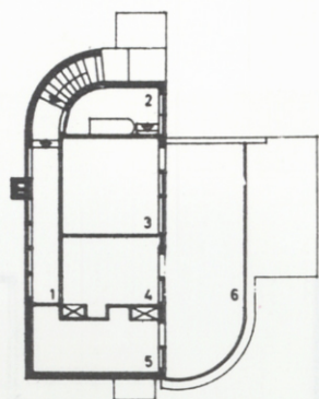
Planta primera.
