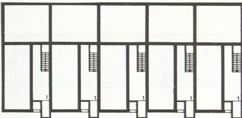
Planta sótano.
