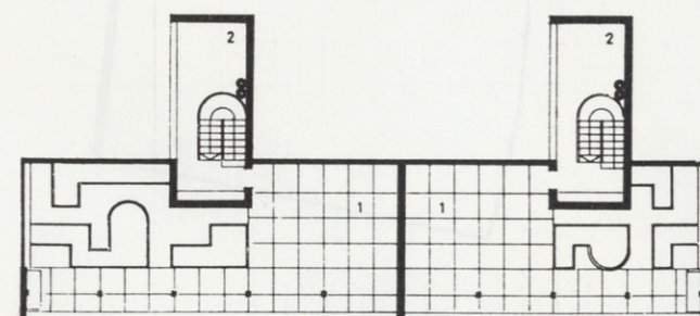
Planta segunda.
