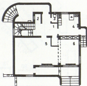
Planta baja.
