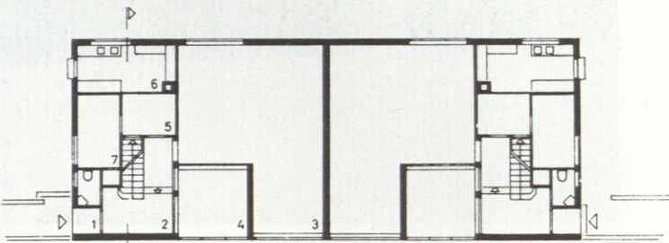
Planta baja.
