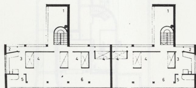
Planta primera.
