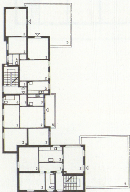
Planta primera.
