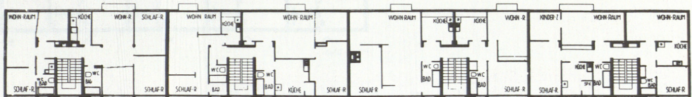
Tercera planta.
