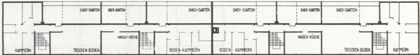
Cuarta planta.
