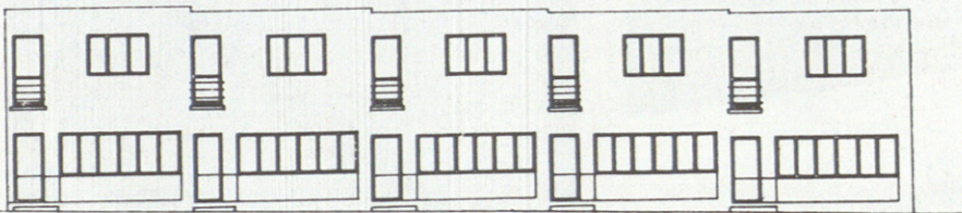
Alzado a jardín.
