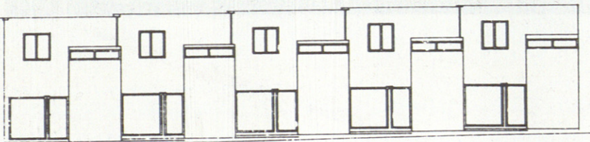
Alzado a calle.
