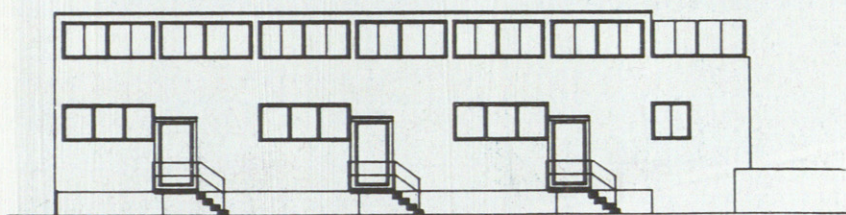
Alzado a calle.
