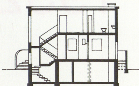
Sección.
