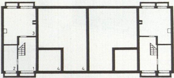
Planta sótano.
