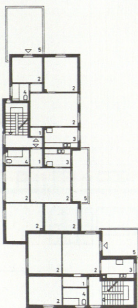
Planta segunda.
