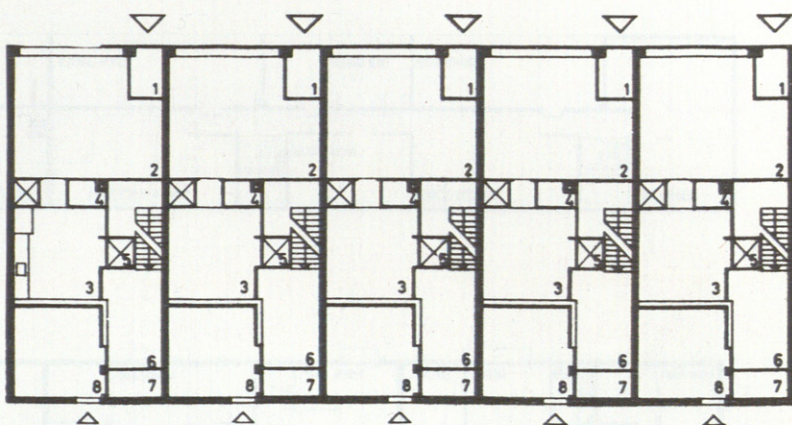
Planta baja.
