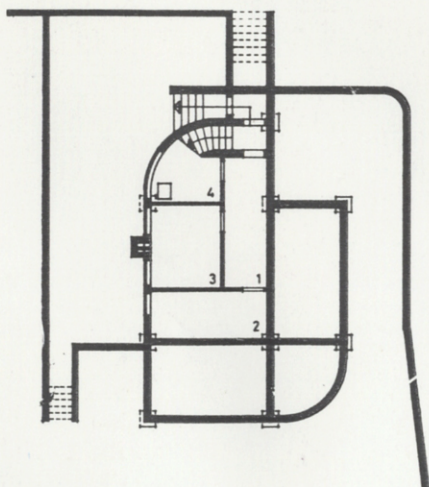
Planta sótano.
