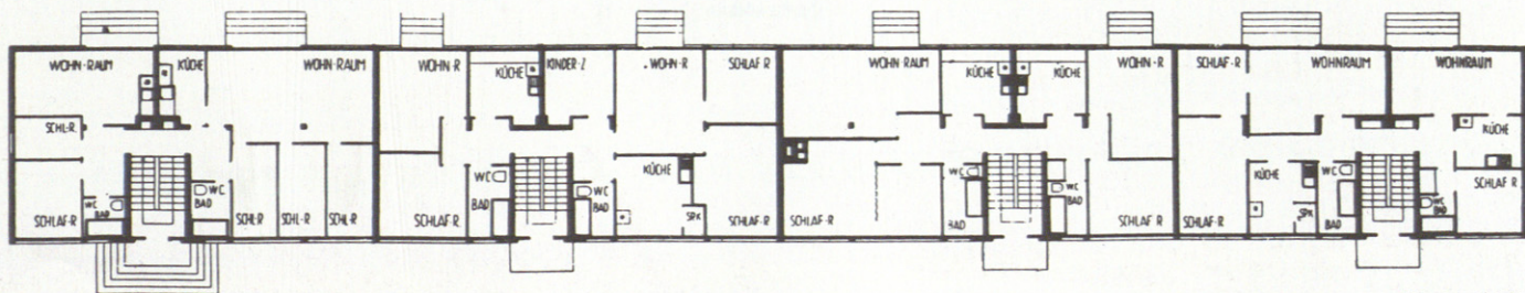
Primera planta.
